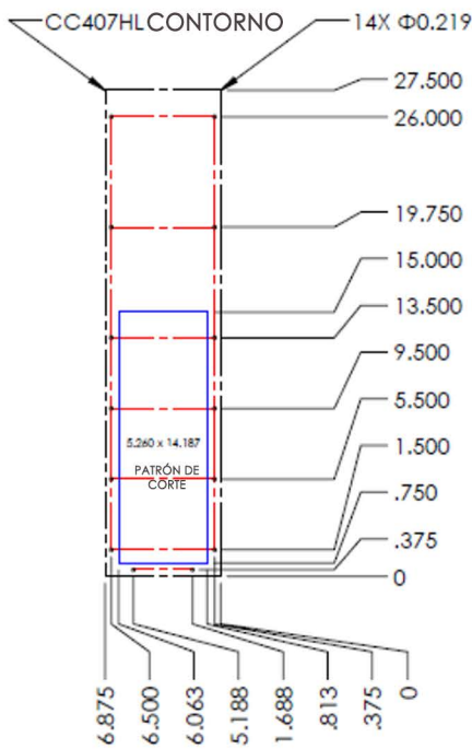
PATRÓN DE AGUJEROS DEL GABINETE (VISTA EXTERNA)
