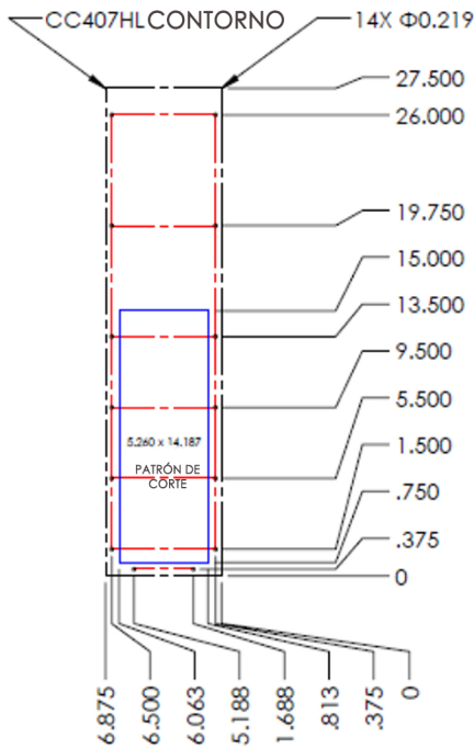
PATRÓN DE AGUJEROS DEL GABINETE (VISTA EXTERNA)
