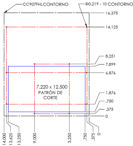
PATRÓN DE AGUJEROS DEL GABINETE (VISTA EXTERNA)
